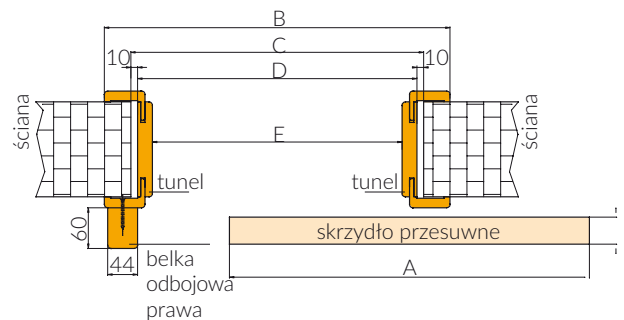
PRZEKRÓJ POZIOMY SYSTEMU PRZESUWNEGO NAŚCIENNEGO Z TUNELEM
