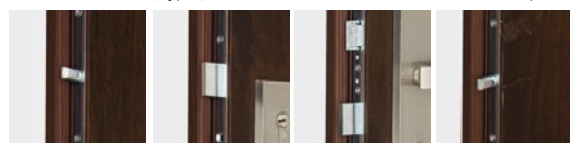
5. zamek czteropunktowy dostosowany pod dwie wkładki patentowe 6. uszczelka w przyldze skrzydła
