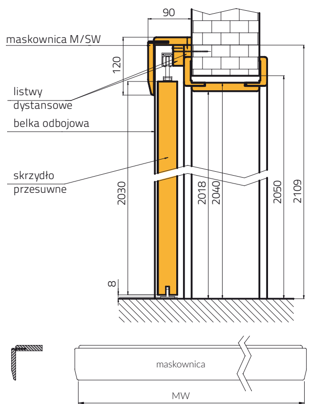
PRZYKŁAD ZASTOSOWANIA SYSTEMU PRZESUWNEGO NAŚCIENNEGO Z TUNELEM
